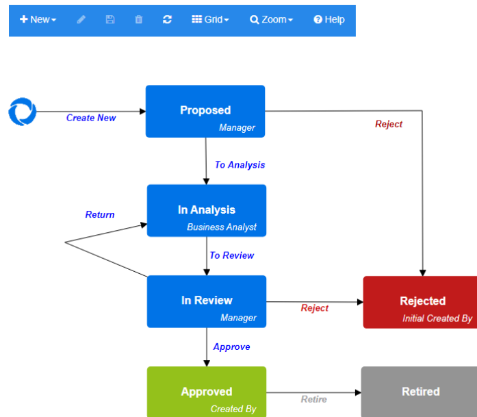
Figura 11-12. Flujo de trabajo para la clase Product_Requirements
