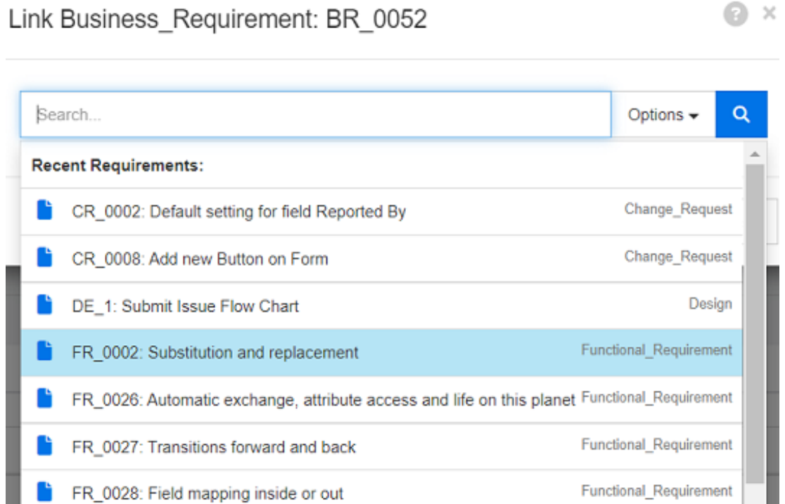
Abbildung 3-7. Klicken Sie in das Feld „Suchen“, um die Anzeige der letzten Anforderungen zu erzwingen.
