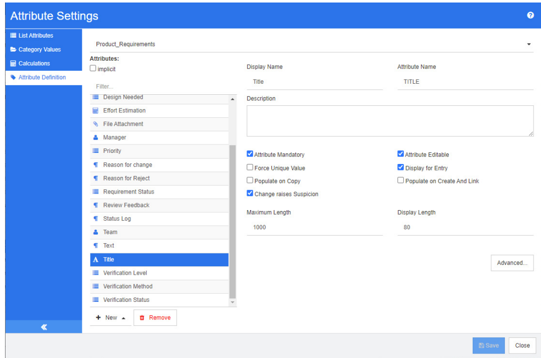
Abbildung 11-1. Alphanumerische Attributdefinition
