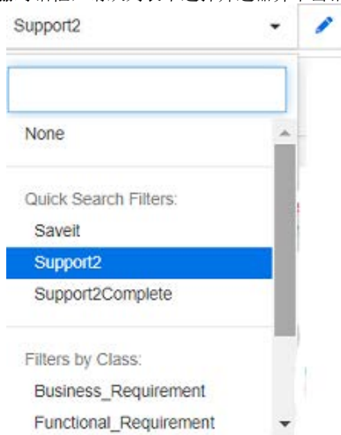
图 4-1. 从文档视图中，选择要编辑的筛选器
