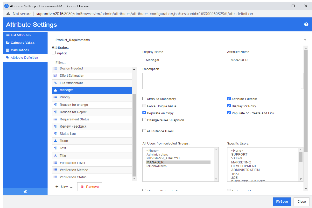
图 11-9. 用户特性定义
