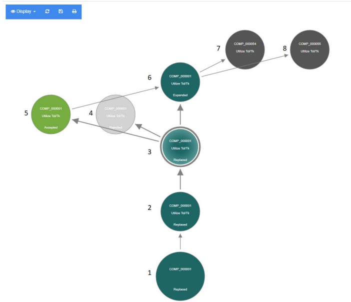
图 3-11. 需求的系谱视图
