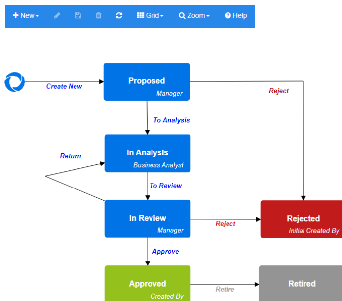
图 11-12. Product_Requirements 类的工作流
